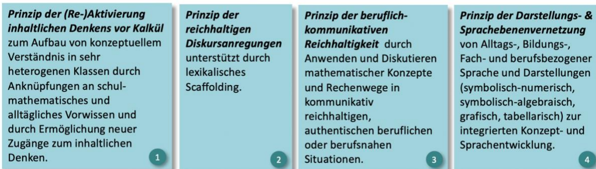
Abb. 1: Vier LaMaVoC-Unterrichtsprinzipien
